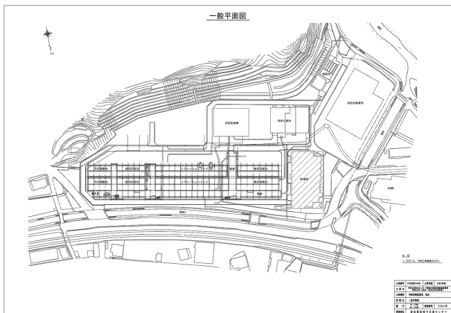
一般平面図
