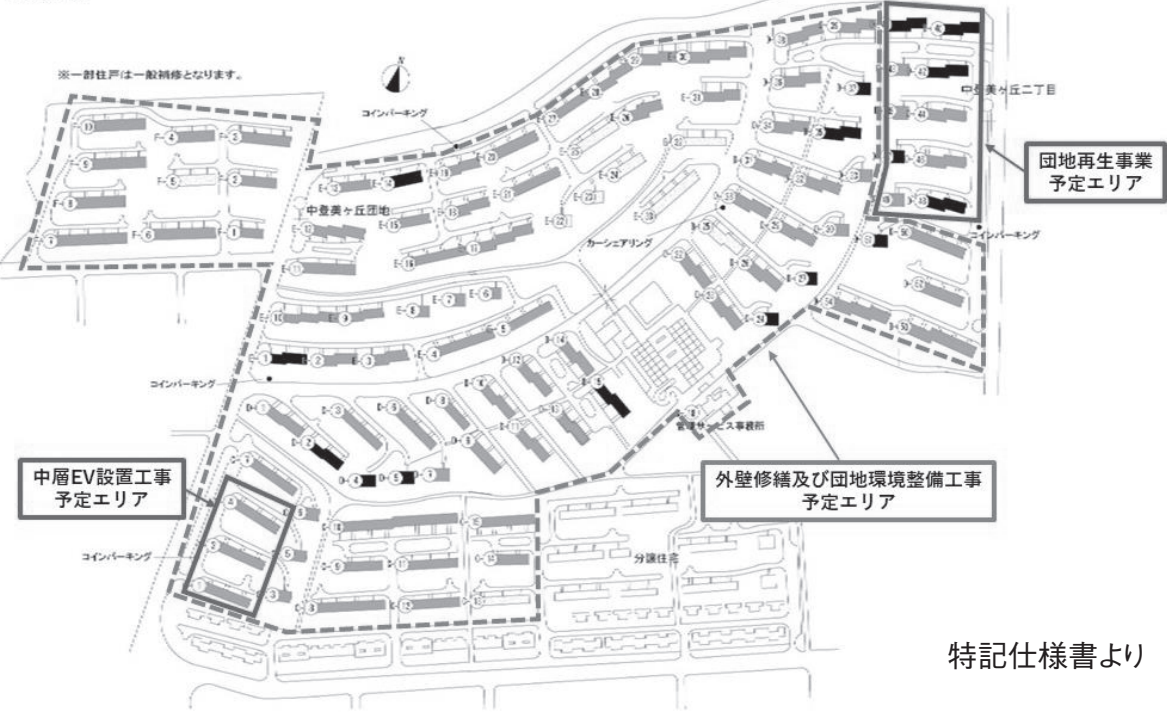
■団地配置図
