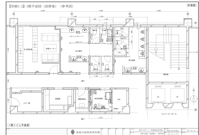
1階平面図(改修後)(参考図)
