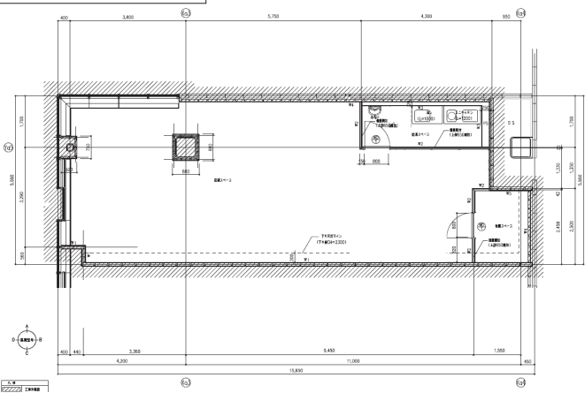
ベルテラスいこま3階A2～304 平面図
