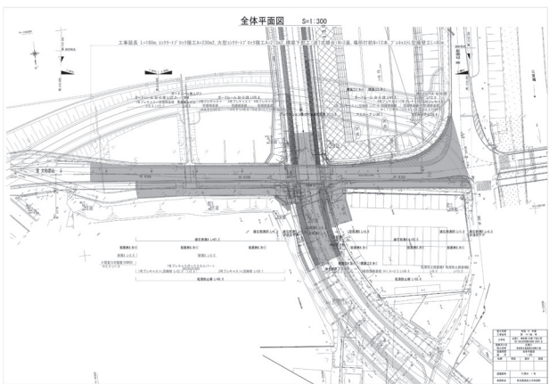
全体平面図(広瀬川無名橋(大場)下部工事)
