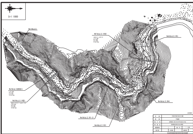
平面図(ゼロ国流域保全総合治山)
