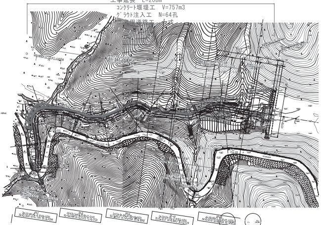
【平面図他】池津川砂防堰堤改築工事
