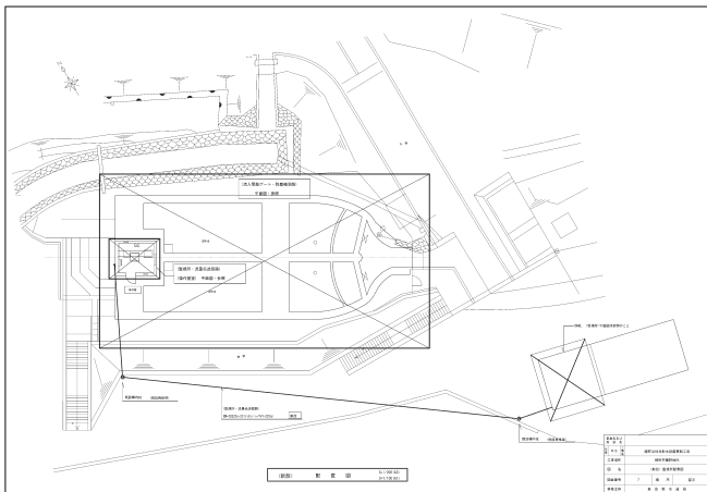
配置図
