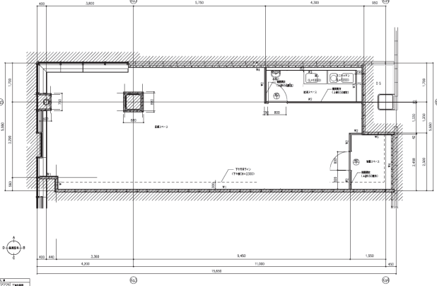
ベルテラスいこま3階A2-304 平面図
