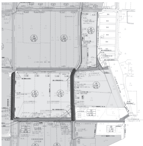
計画平面図
