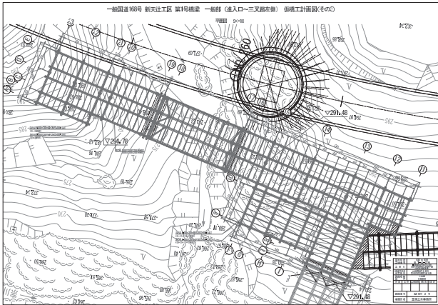
第1号橋梁進入仮橋工事計画図
