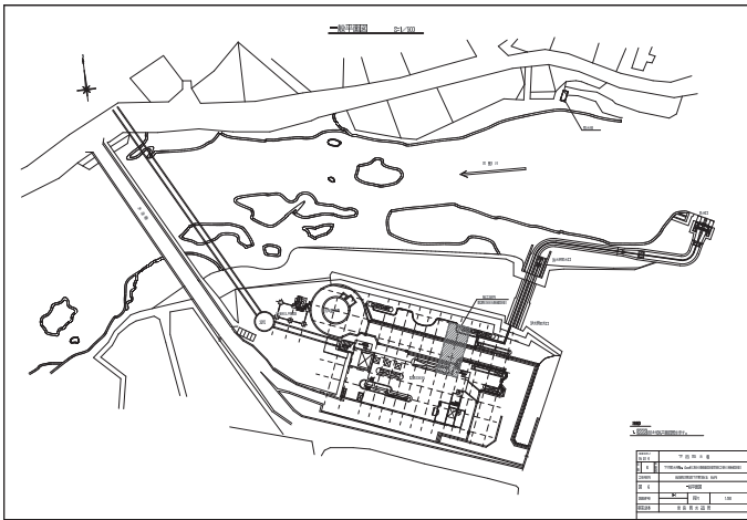
一般平面図
