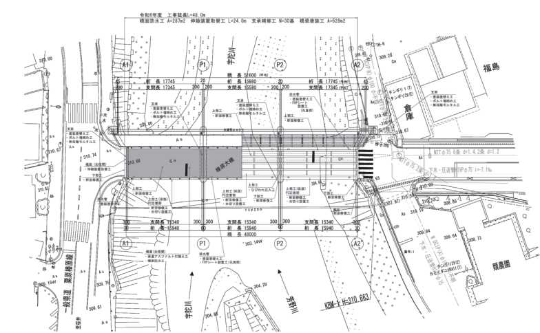
補修工一般図
