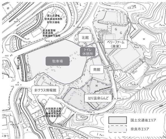
施設配置図
