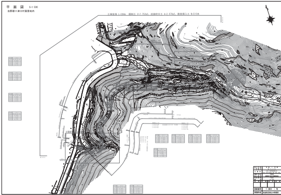
大谷谷管理用道路設置工事平面図
