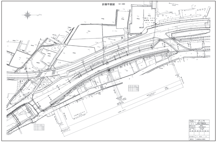
計画平面図
