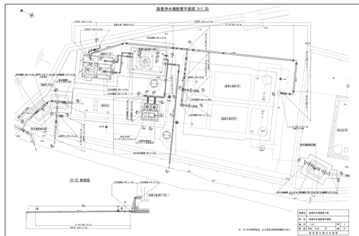
阪巻浄水場配管平面図
