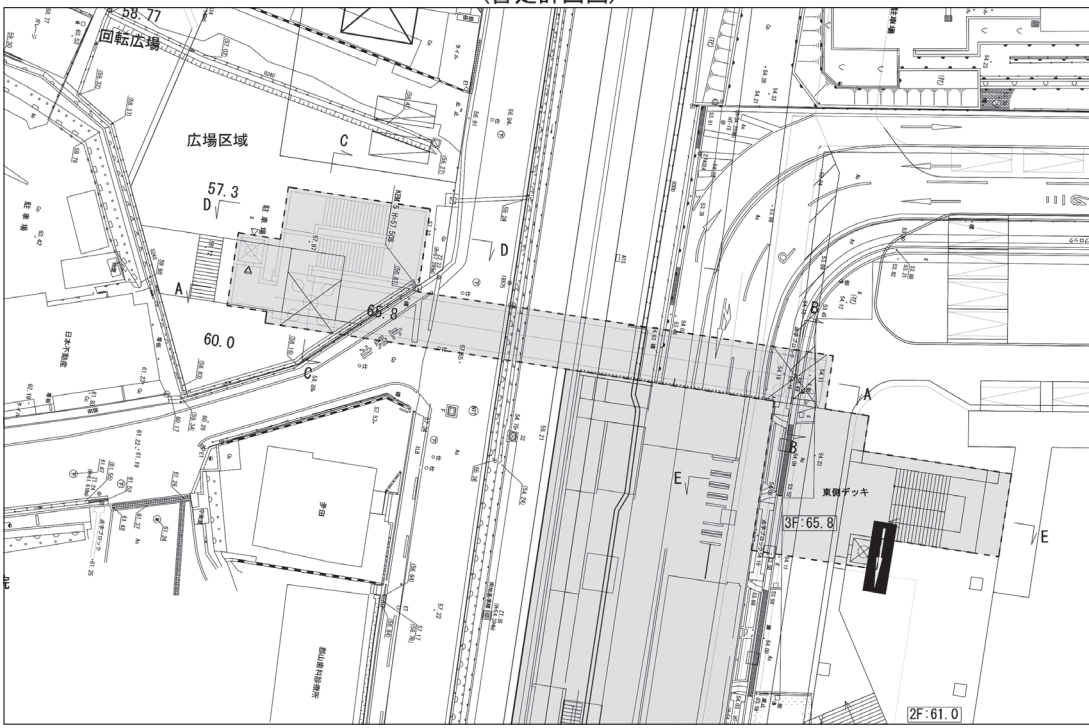
自由通路構造一般図 S=1:400(A3) (暫定計画図)
