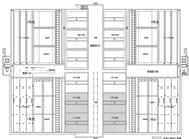
広域平面図
