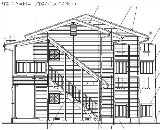
施設の立面図4(道路から見て右側面)
