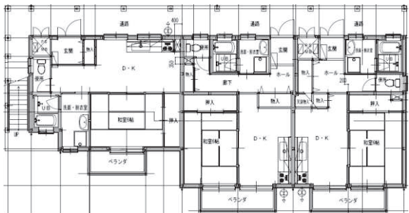
施設の1階平面図
