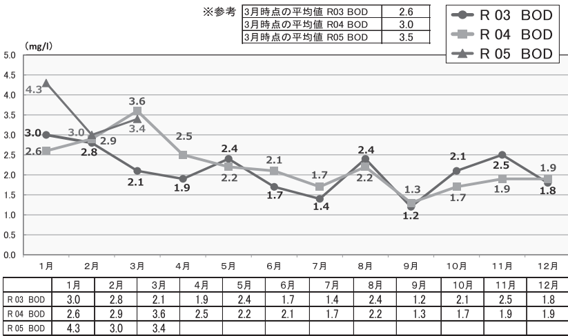
R03 - R04 - R05 大和川本川8地点水質平均値比較
