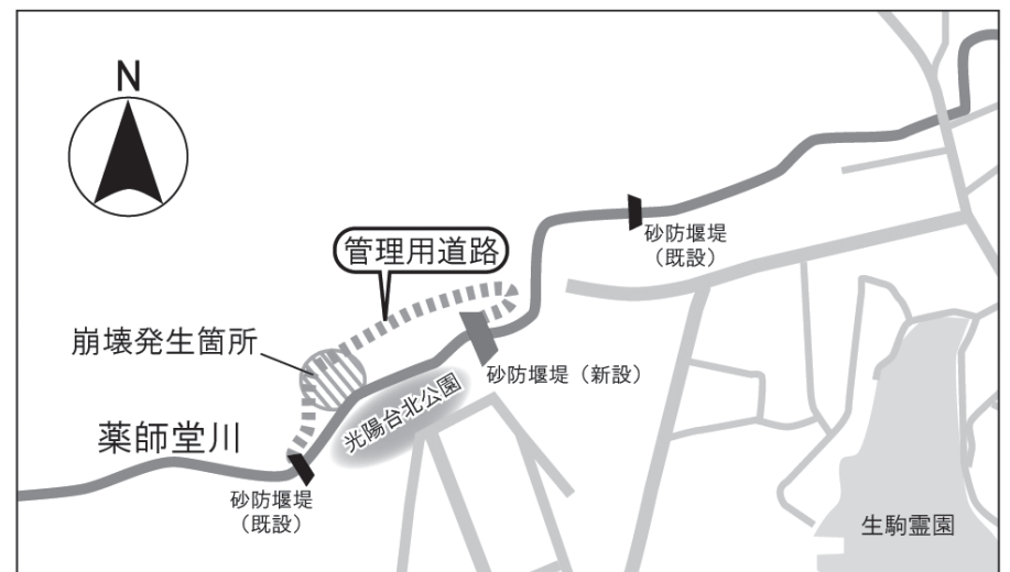
砂防堰堤管理用道路の法面などを整備する
