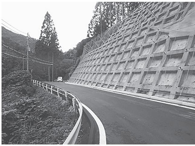
工事が完了したⅡ-1工区
