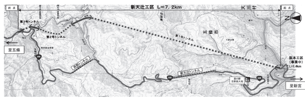
新天辻工区概略平面図
