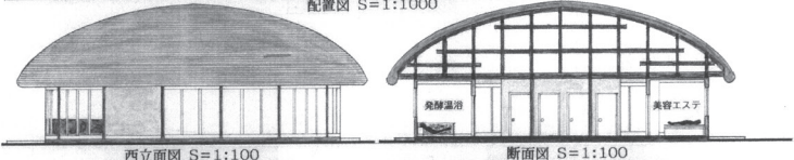
西立面図 S=1:100
