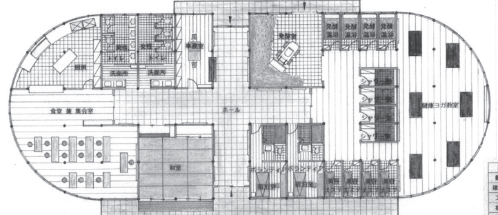
平面図 S=1:100
