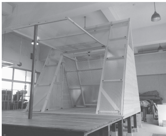
実際に制作されたヨガハウス
