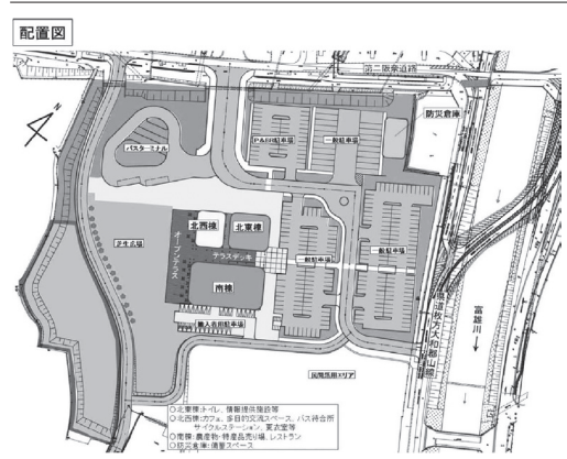
配置図
