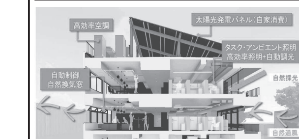
技術研究所管理棟のZEB化改修の採用技術
